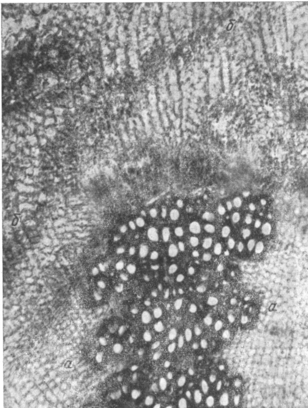
Рис. 3. Поперечный срез корневища
