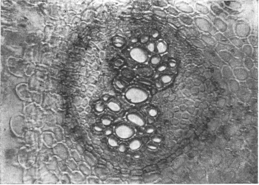
Рис. 2. Первичное строение корня (поперечный срез)
