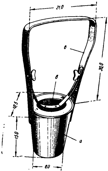
Рис. 1. Ручной садовый лункокопатель. Объяснения — в тексте
